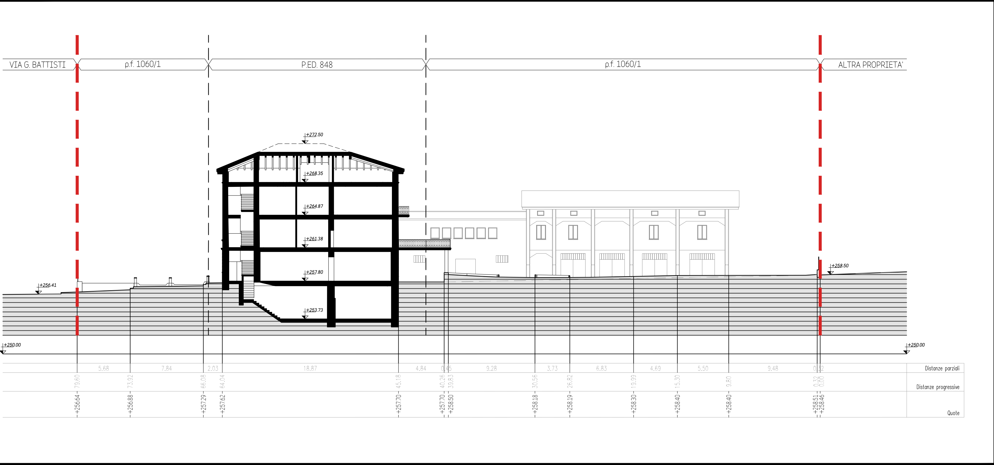
SEZIONE B-B
